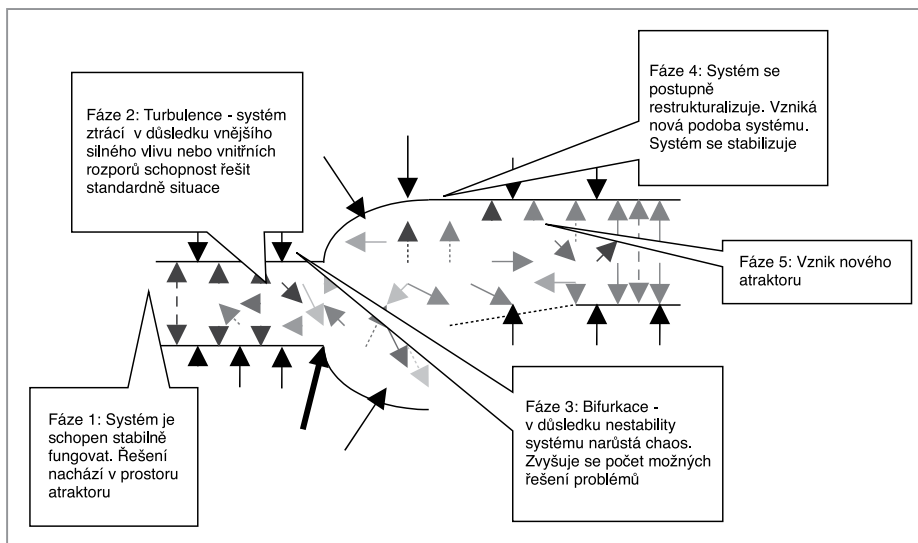
Graf 2 Bifurkační bod v systémové teorii
